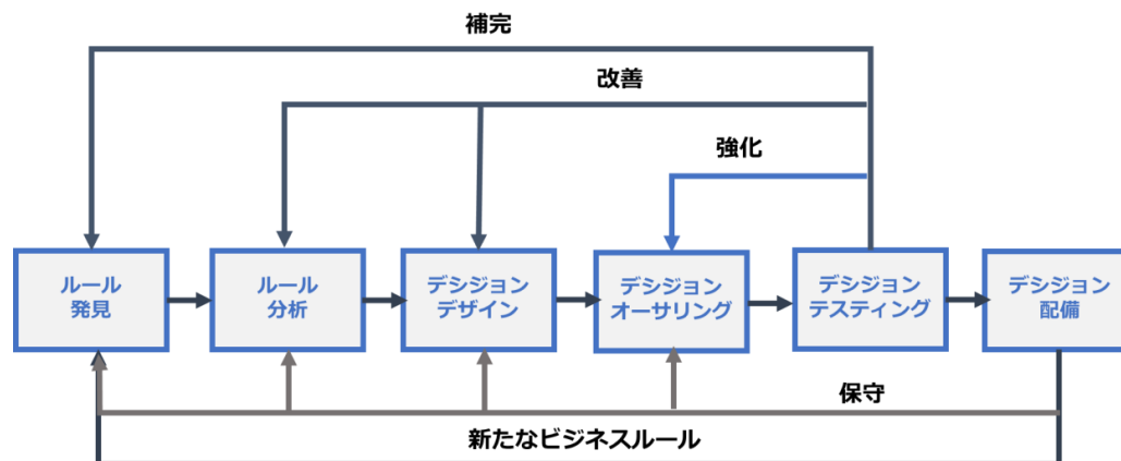
図 9 意思決定ライフサイクル・フェーズ
