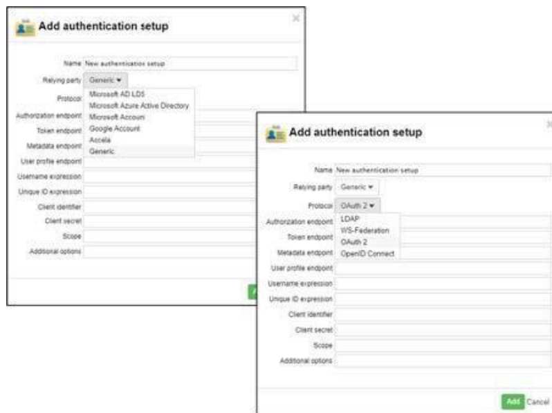
図 13 認証プロバイダと設定
