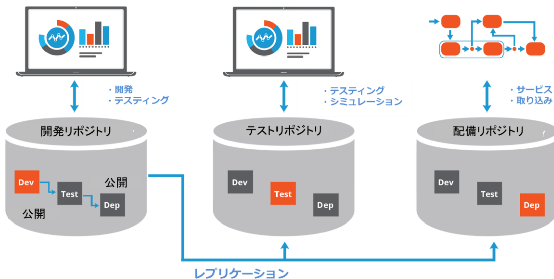
図 10 リリースのレプリケーション
