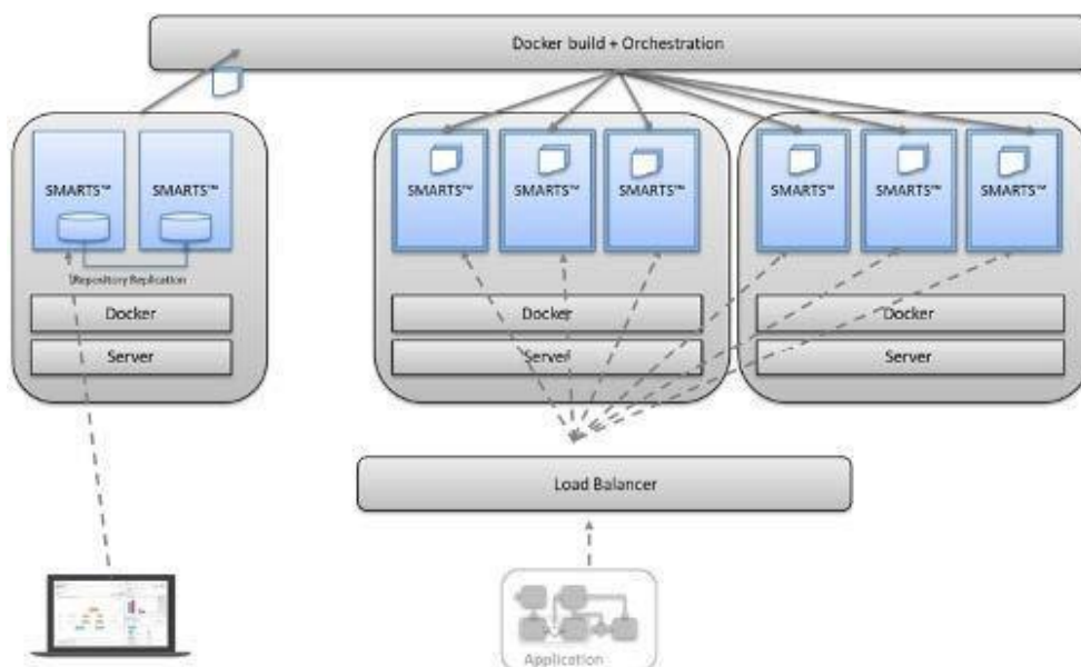
図 12 デプロイにオーケストレーションツールを活用
